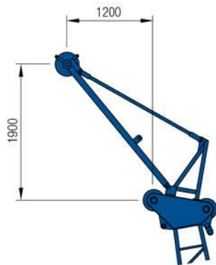
Falchetto ausiliario 3 ton. Auxiliary jib 3 ton.
